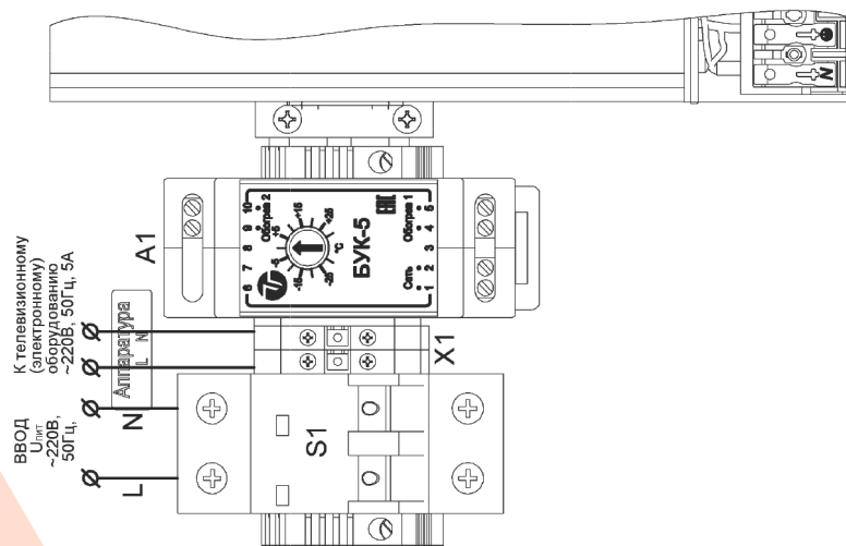
Рис.2. Подключение термощафа
